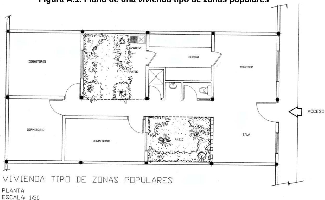
Figura A.1. Plano de una vivienda tipo de zonas populares
