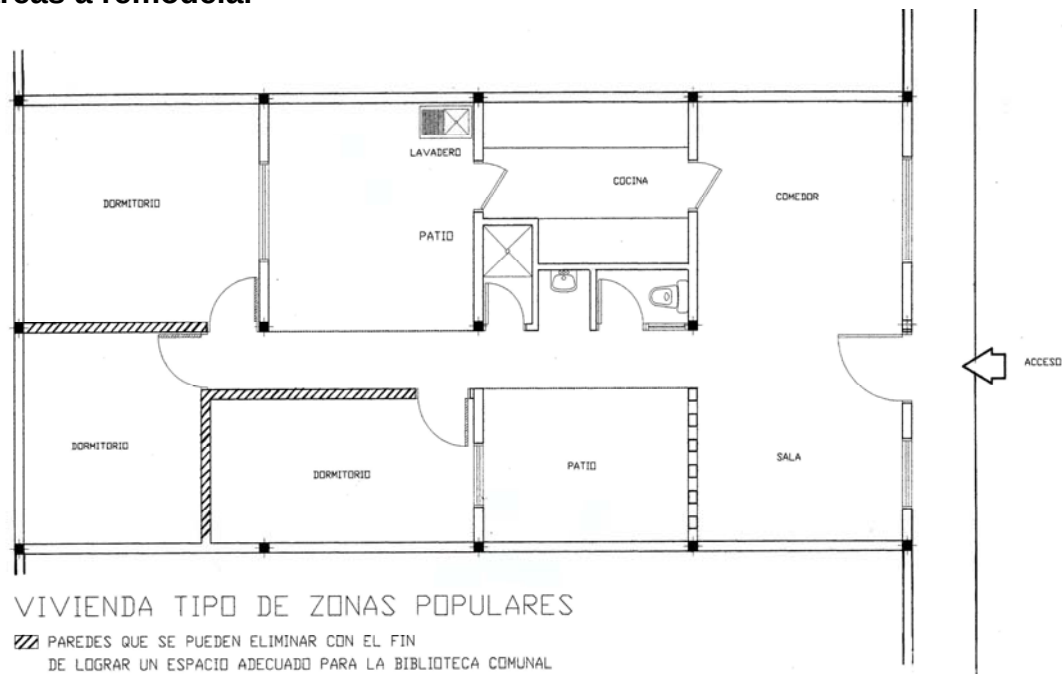
Figura A.2. Plano de una vivienda tipo de zonas populares con la indicación de áreas a remodelar
