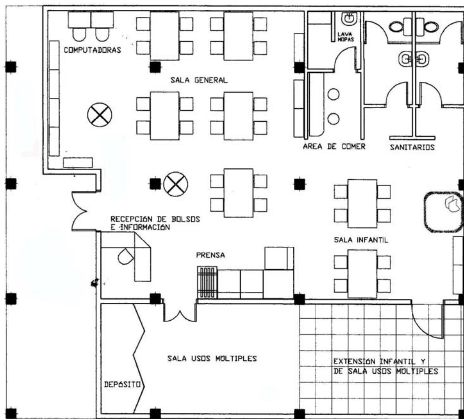
BIBLIOTECA COMUNAL TIPO ESCALA 1:50
