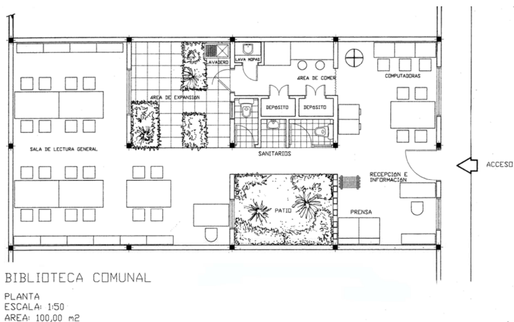
Figura A.3. Plano de la propuesta para la Biblioteca Comunal
